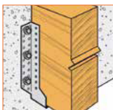
GSE : Fixation sur support rigide BÉTON ou ACIER
